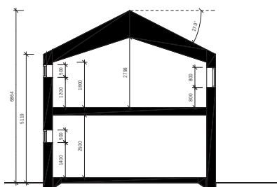
↑ Sektion
