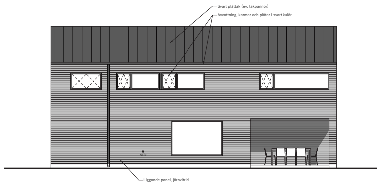
↑ Fasad långsida
