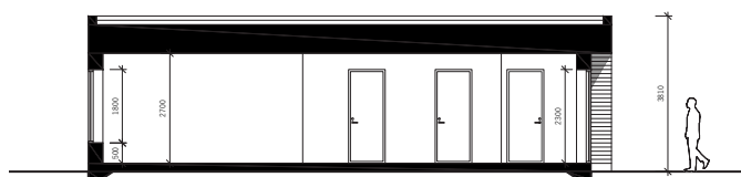
↑ Sektion A-A
