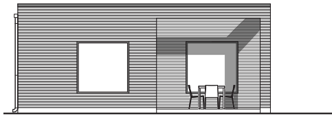
↑ Fasad kortsida
