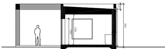
↑ Sektion B-B
