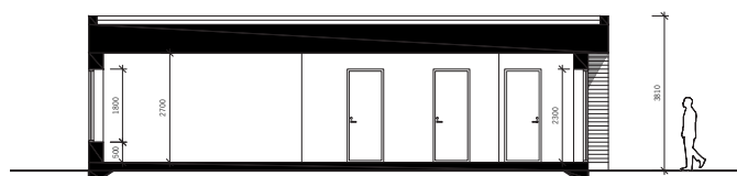
↑ Sektion A-A
